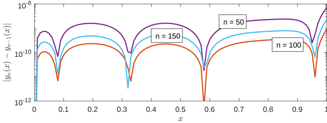
Figura 7.4: Diferença nas imagens de duas aproximações consecutivas para o Exemplo 7.1, com n = 50, 100, 150 , resultante da aplicação do método tau e operando com as matrizes de mudança de bases.
